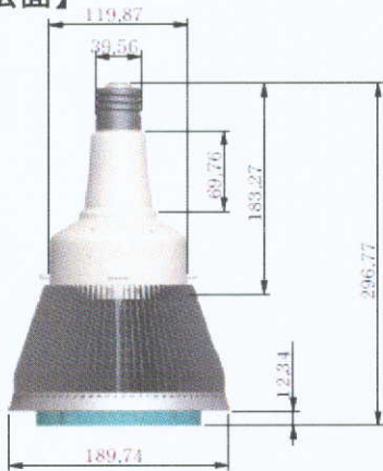
【寸法面】
